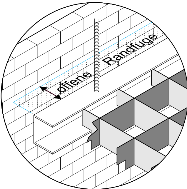
Offene Randfuge (Variante 1) U.- Profil als Rasterabschluss halbverdeckte Montage
