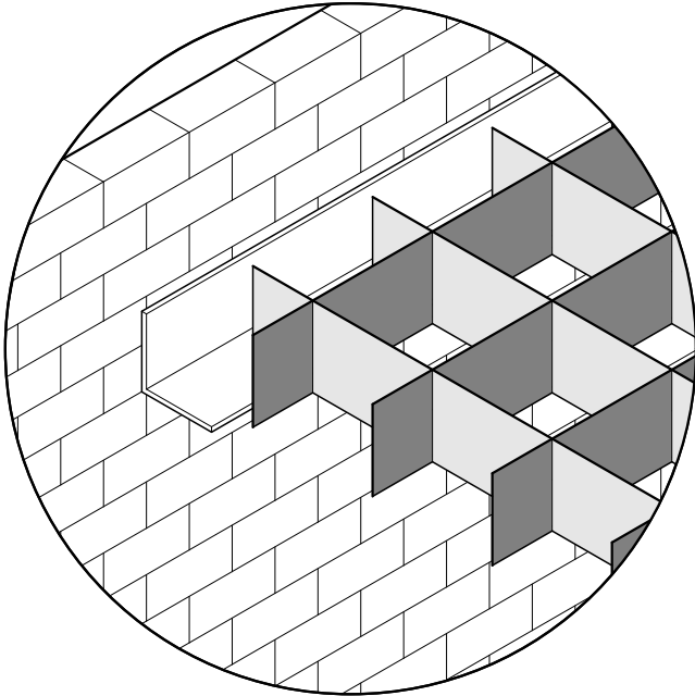
L - Winkel, stumpf aufgelegt
