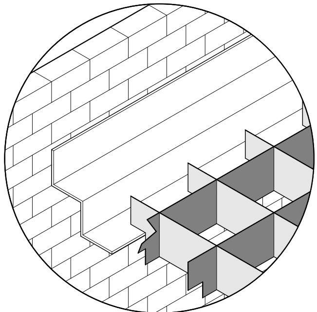
Stufenwinkel, halbverdeckte Montage
