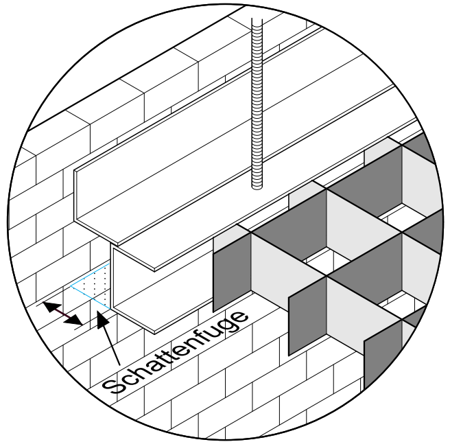
Abgedeckte Randfuge (Variante 2) U.- Profil als Rasterabschluss und Befestigung über zweiteilige, verschiebbare Randwinkel halbverdeckte Montage
