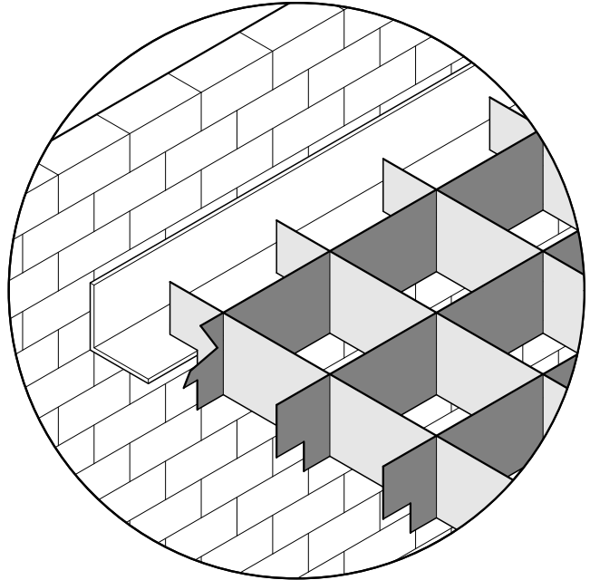
L - Winkel, halbverdeckte Montage
