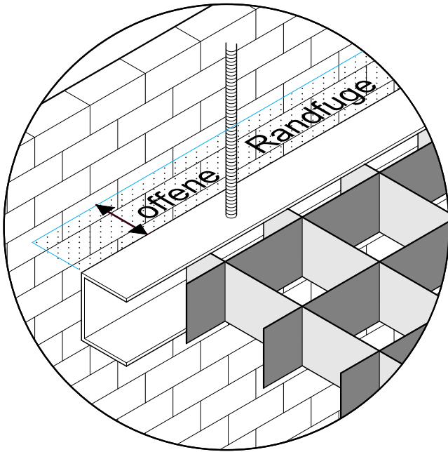
Offene Randfugen U.- Profil als Rasterabschluss
