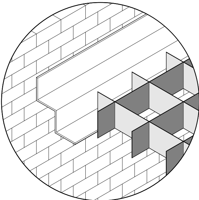
Stufenwinkel, stumpf aufgelegt
